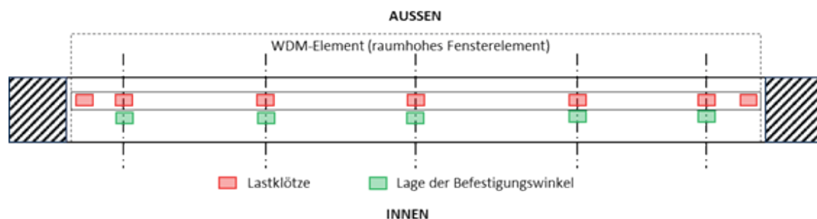
1b) Schematische Positionierung der Lastklötze (Ausführung WINDOWMENT®: raumhohes Fensterelement)
