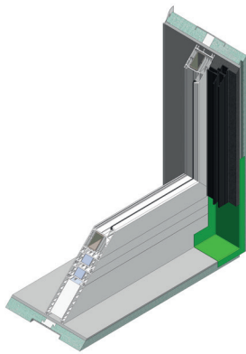
Abdichtung durch den werkseitig ausgeführten Abdichtungs-lappen
