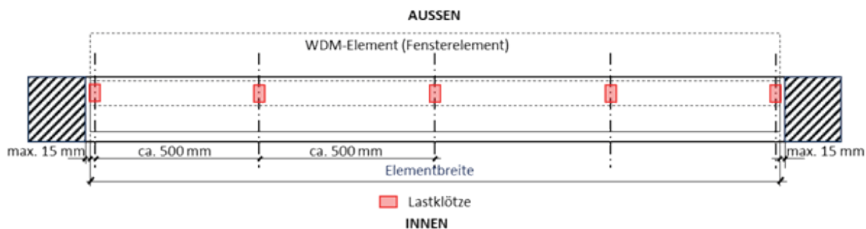
1c) Schematische Positionierung der Lastklötze (Ausführung WINDOWMENT®-Fensterelement)
