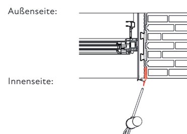
Schritt 2: Einbringung des nachdruckfreien PU-Schaums von innen
