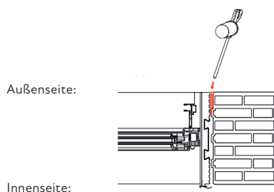
Schritt 1: Einbringung des nachdruckfreien PU-Schaums von außen
