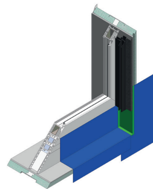
Schematische Darstellung der bauseitigen Abdichtung, z.B. mittels Flüssigkunststoff
