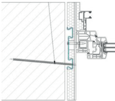
Befestigung durch G-Schiene mittels Rahmenanker im Mauerwerk
