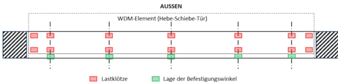
1a) Schematische Positionierung der Lastklötze (Ausführung WINDOWMENT®: HST-Element)
