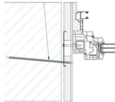
Befestigung durch C-Schiene mittels Rahmenanker im Mauerwerk
